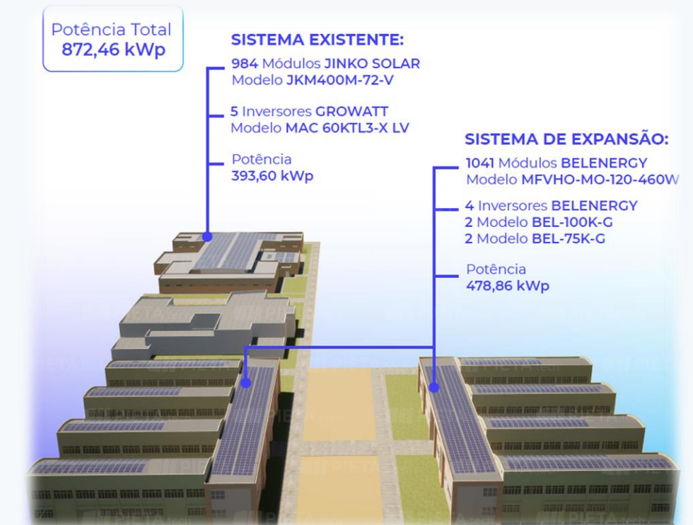
Esquematização dos sistemas de energia solar fotovoltaica no CRES.
